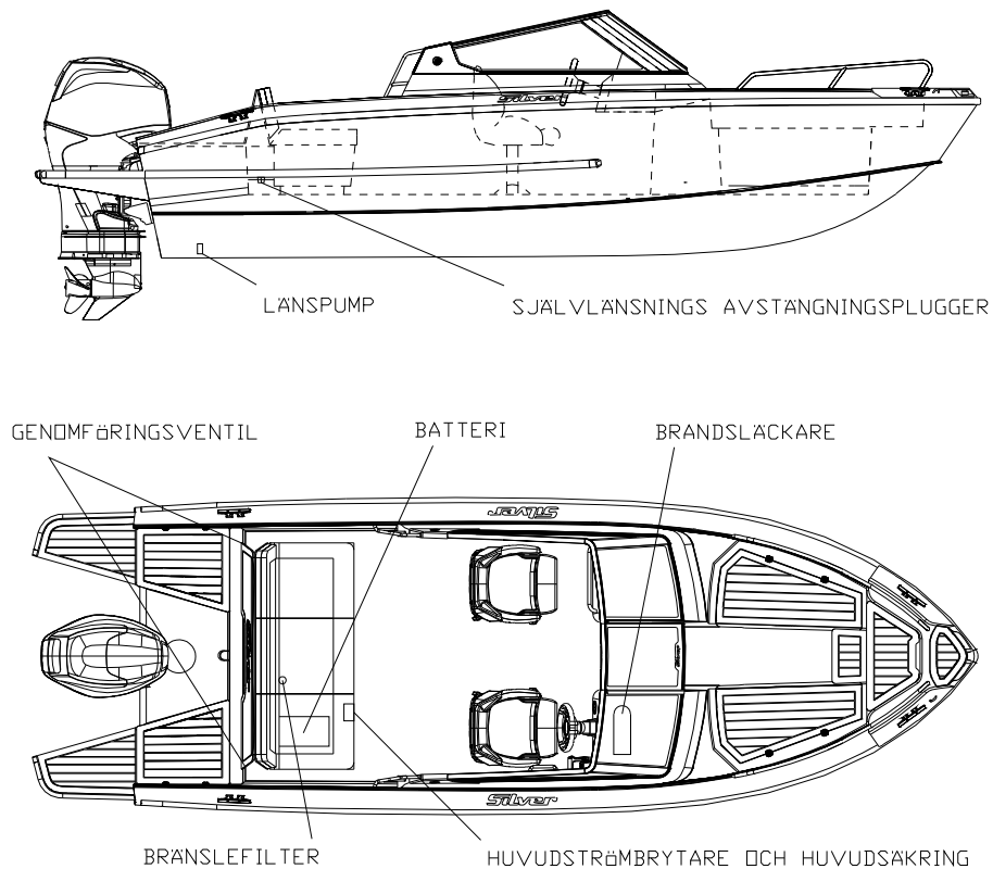
110 Bild 5. Placering av bordgenomföringar, avstängningsventiler och länsumpar.
