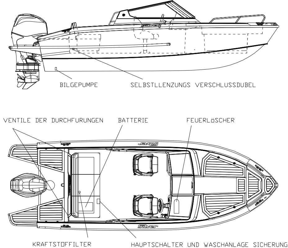
236 Abbildung 5. Lage der Durchführungen und Verschlussventile sowie der Bilgepumpen.
