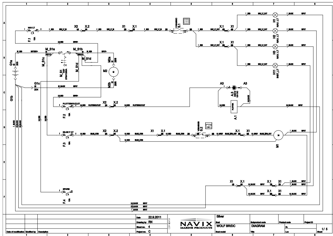
Kuva 6. Sähkökaavio
