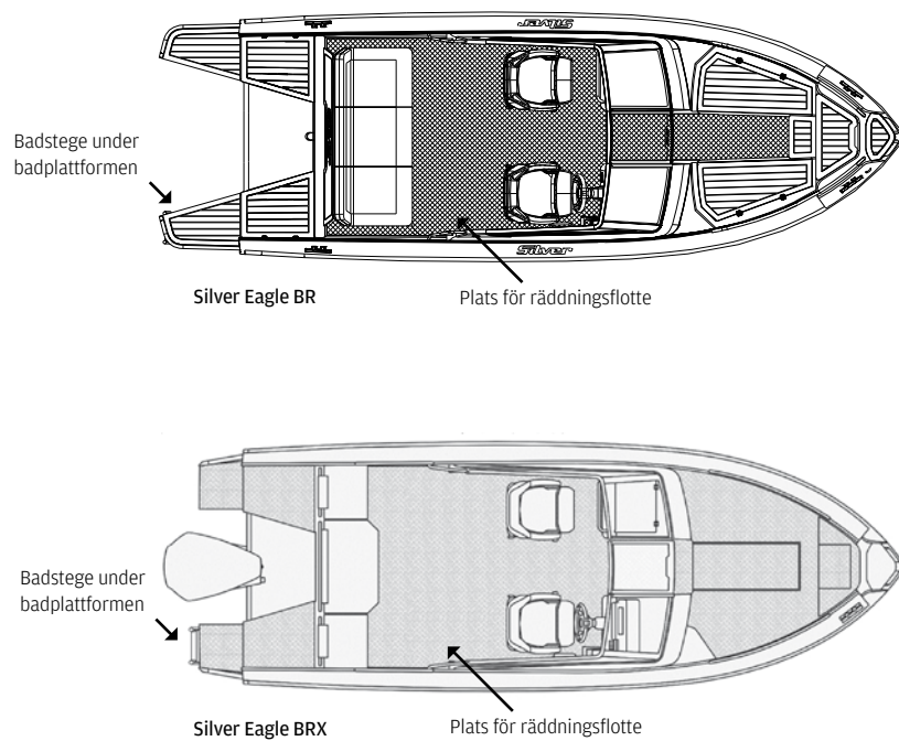
Bild 4. Placeringen av simstege och halkskydd, samt rekommenderad placering för räddningsflotte.
