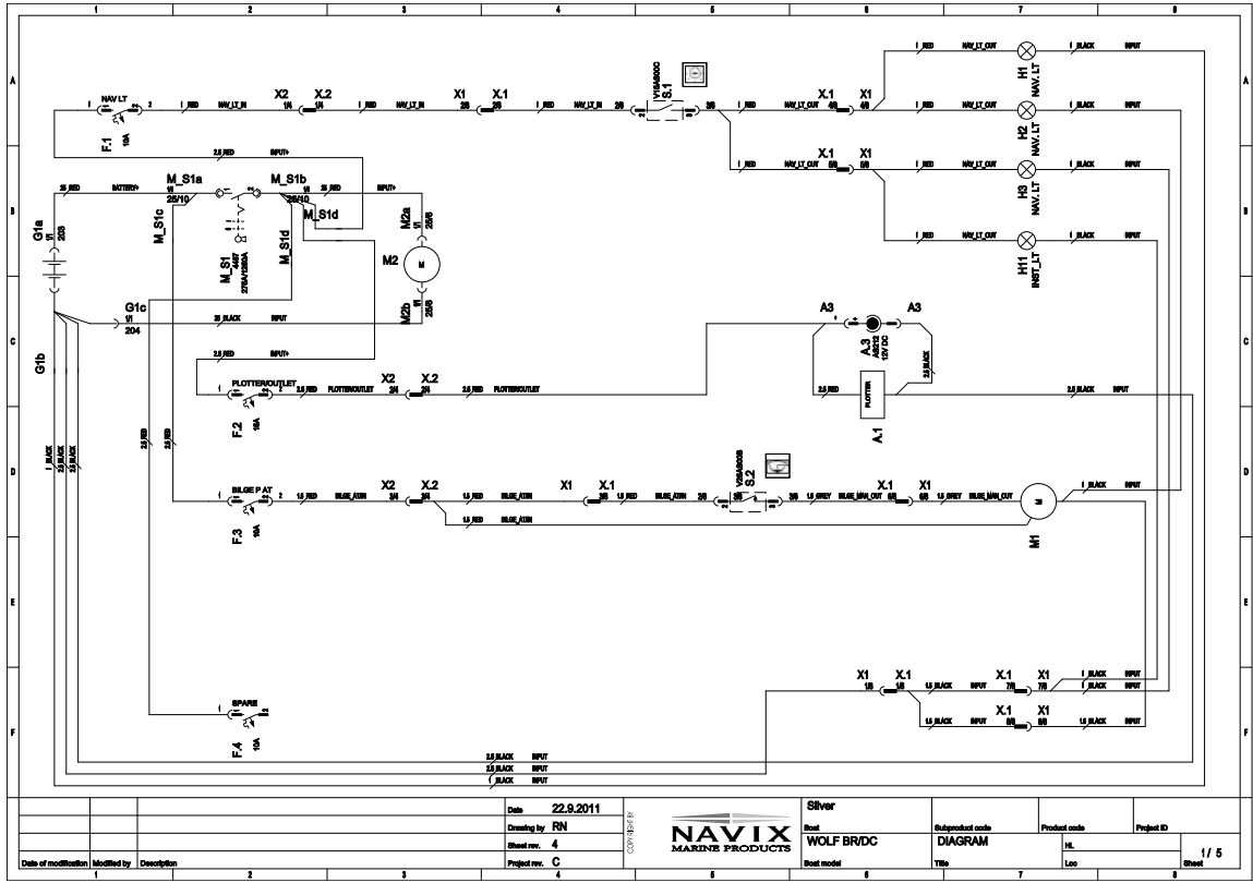
Bild. 6 Elschema
