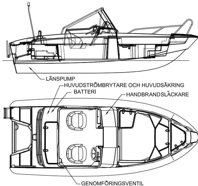
Bild 5. Placering av bordgenomföringar, avstängningsventiler och länsumpar.
